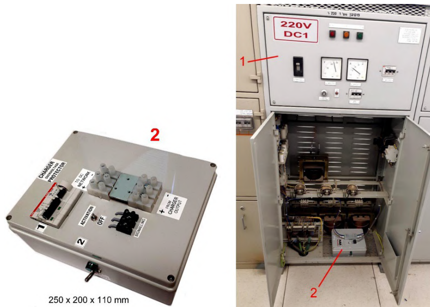
Fig. 21. Charger disconnection module
